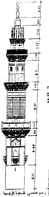
رسم هندسي للمنارة الرئيسية.
