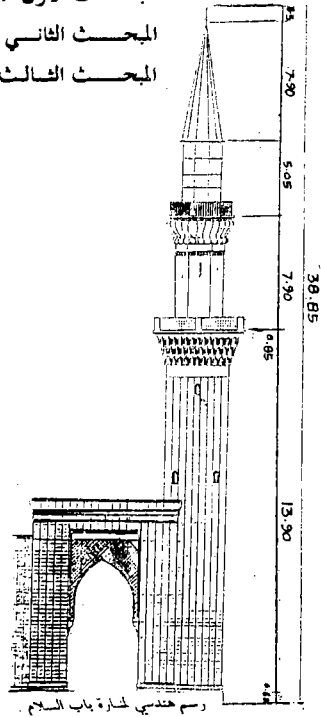
رسم هندسي لمنارة باب السلام.
