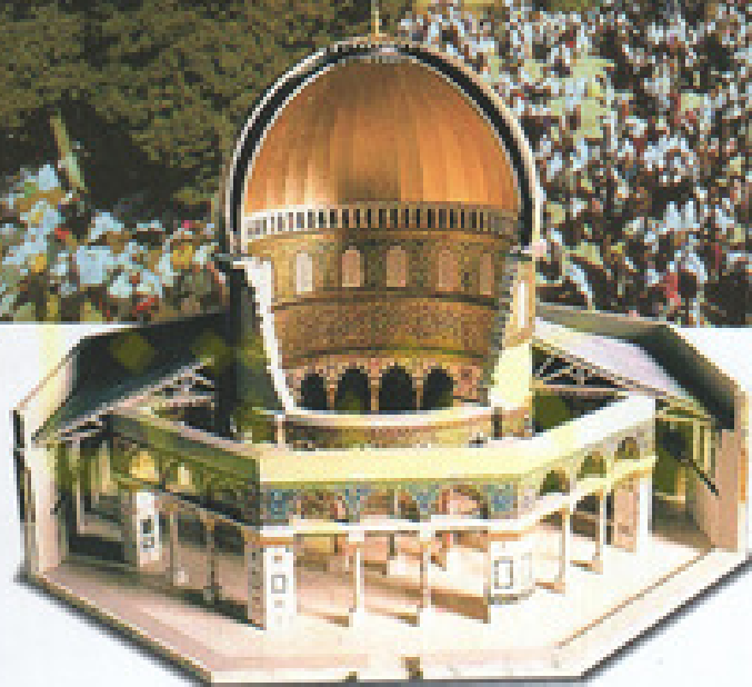
● مقطع لقبية الصخرة
